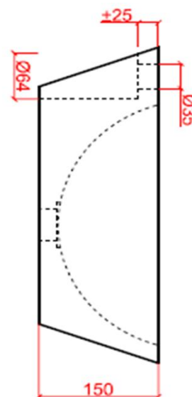
zijaanzicht / vue de côté
