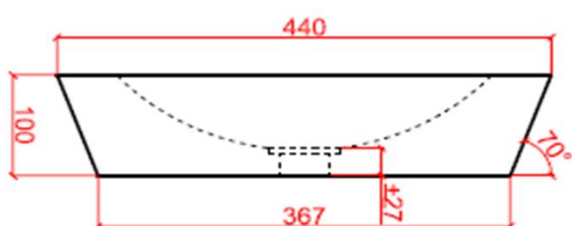
vooraanzicht / vue de face
