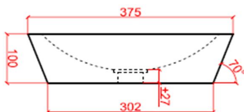
vooraanzicht / vue de face
