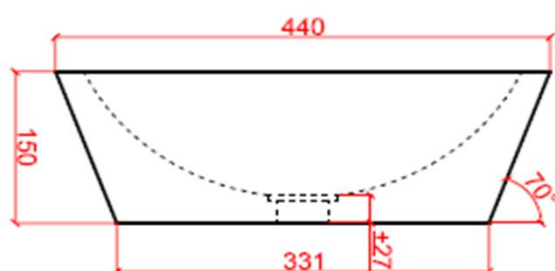
vooraanzicht / vue de face
