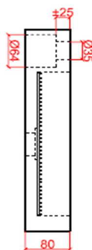
zijaanzicht / vue de côté
