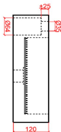
zijaanzicht / vue de côté
