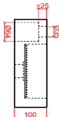
zijaanzicht / vue de côté
