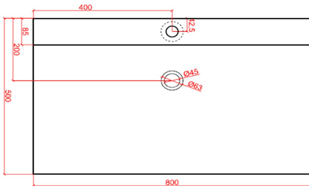
bovenaanzicht / vue d'en haut
