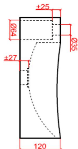
zijaanzicht / vue de côté
