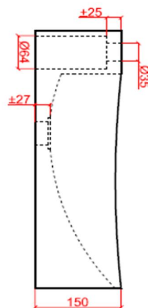
zijaanzicht / vue de côté
