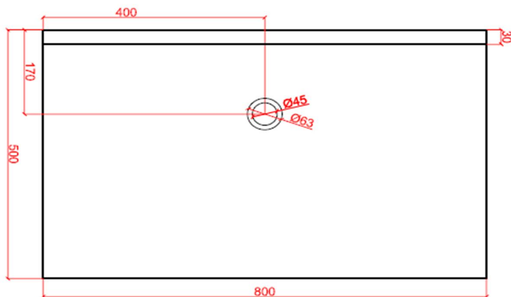
bovenaanzicht / vue d'en haut
