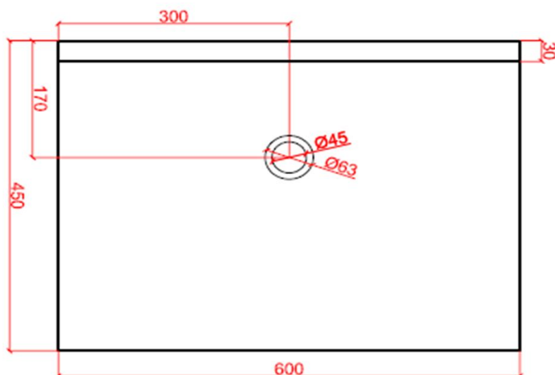
bovenaanzicht / vue d'en haut
