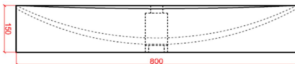
vooraanzicht / vue de face
