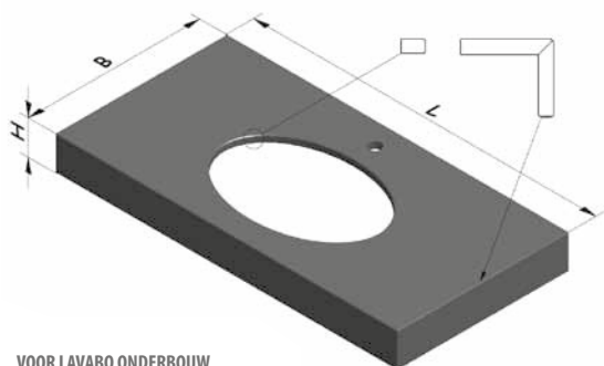
VOOR LAVABO ONDERBOUW POUR VASQUE SOUS-ENCASTRÉE
